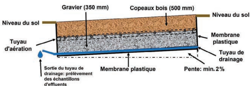
FIGURE 1 : COUPE TRANSVERSALE D'UNE SOP MUNIE D'UN SYSTÈME D'AÉRATION
